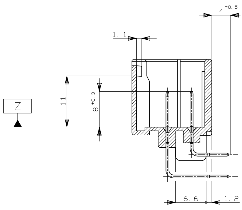
B-B
