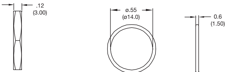
O - RING
