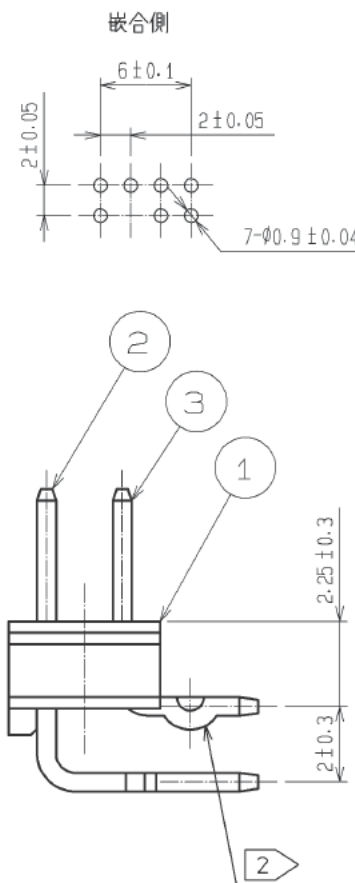
推奨基板寸法図(2:1)
