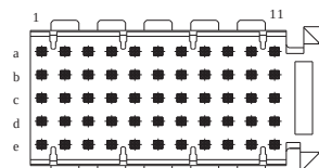
Bestückungsplan - contact layout
