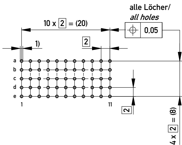
Lochbild für Leiterplatte (Bestückungsseite)
