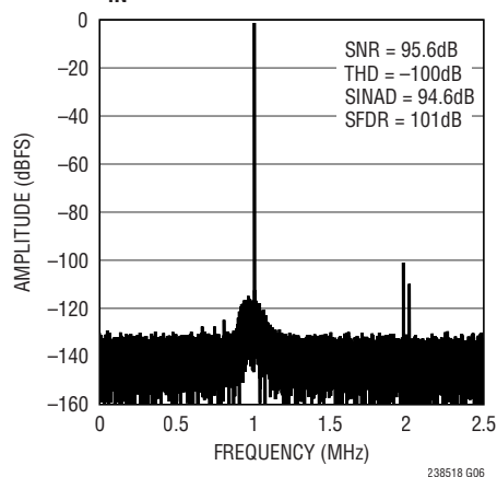
32k Point FFT f_{\text{SAMPL}} = 5\text{Mps} , f_{\text{IN}} = 1\text{MHz}
