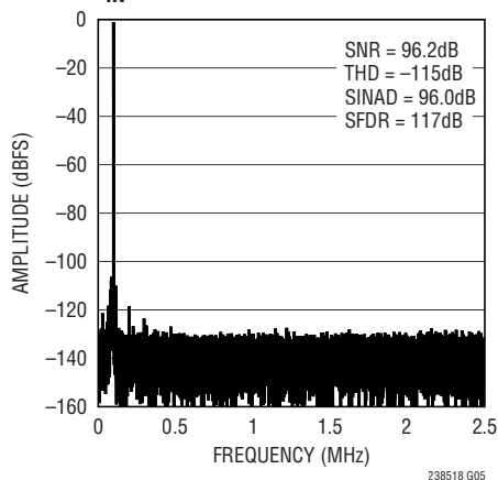
32k Point FFT f_{\text{SAMPL}} = 5\text{Mps} , f_{\text{IN}} = 100\text{kHz}
