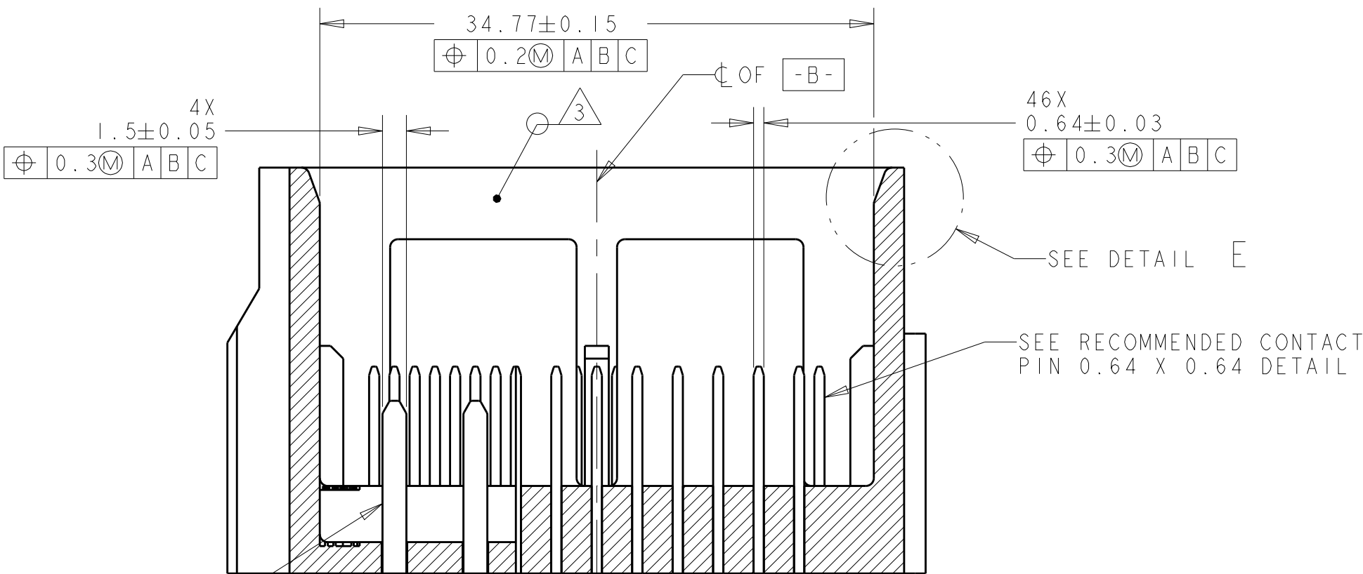
SECTION A-A
