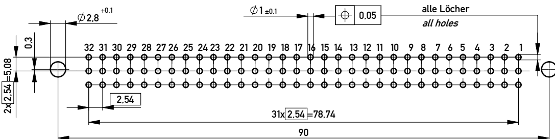
Leiterplatten-Lochbild / PCB drillhole pattern
