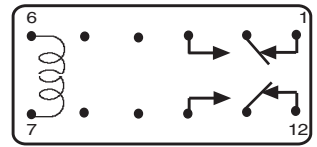
219XBP DPDT
