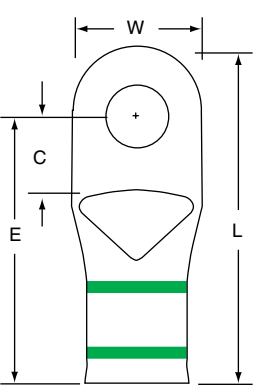
MC1-516RX
