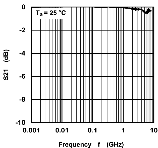
Fig. 9.1 S_{21} - f
