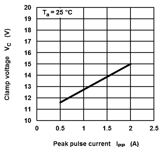
Fig. 8.1 V_C - I_{PP}
