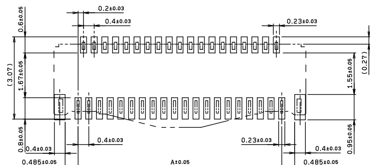
基板取付寸法 MOUNTING LAYOUT
