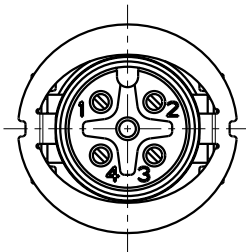
4pol A-Codierung (Steckseite) 4pole A-coding (Plug-in side)
