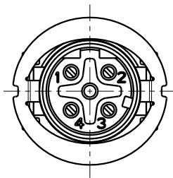
4pol D-Codierung (Steckseite) 4pole D-coding (Plug-in side)
