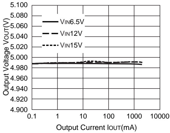
R1224N502M L=27μH
