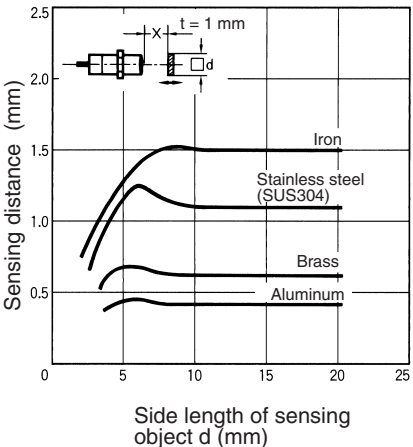
E2E-X1R5E/V E2E-X1R5Y
