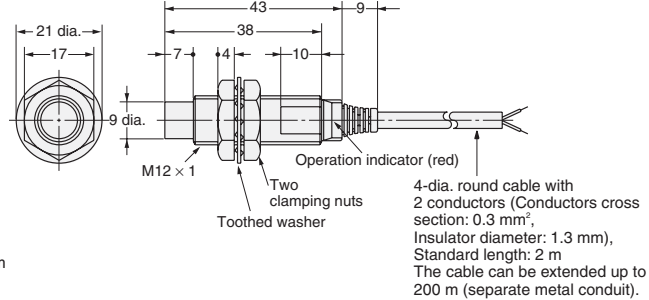
Fig. 11 : E2E-X5MY□
