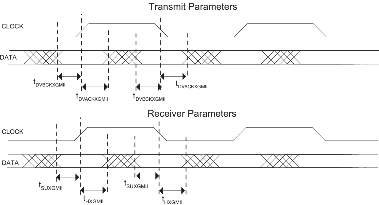
Figure 3-8. XGMII Parameters
