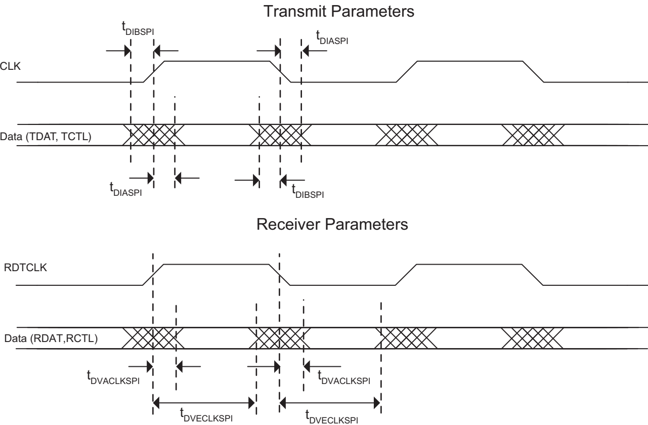
Figure 3-6. SPI4.2 Parameters
