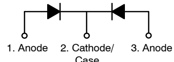
Schottky Diode
