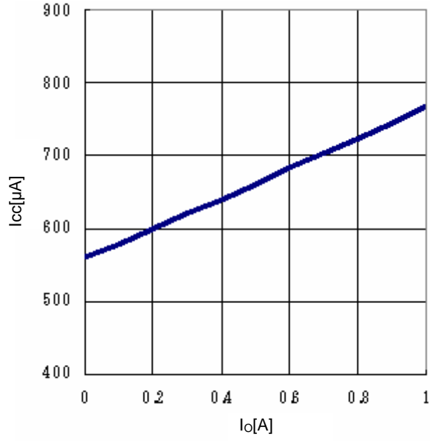
Fig.20 I_o - I_{cc}
