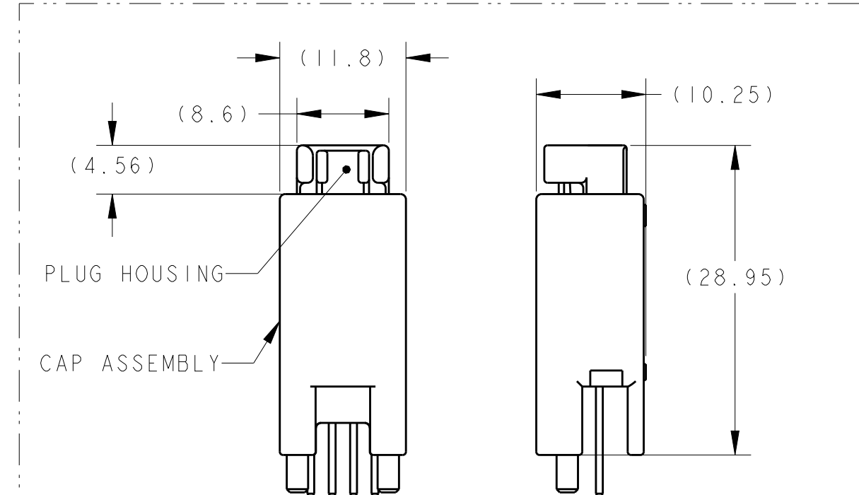
CAP ASSEMBLY & PLUG HOUSING ENGAGEMENT VIEW キャップアセンブリ&プラグハウジング嵌合状態図
