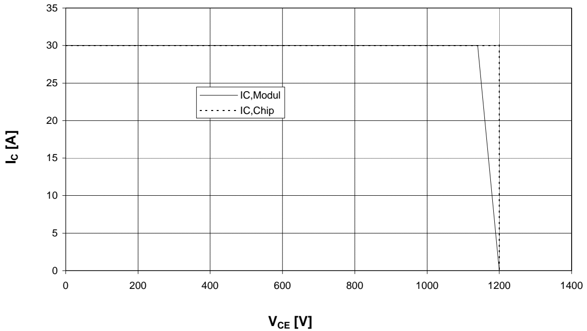
Sicherer Arbeitsbereich Wechselr. (RBSOA) I_C = f(V_{CE}) Reverse bias safe operating area Inverter (RBSOA) T_{vi} = 125^\circ\text{C} , V_{GE} = \pm 15\text{V} , R_G = 47\ \text{Ohm}
