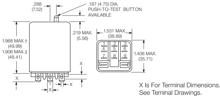
KUP top flange case
