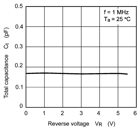
Fig. 7.3 C_t - V_R
