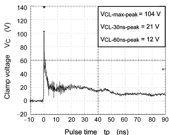
Fig. 10.1 +8 kV
