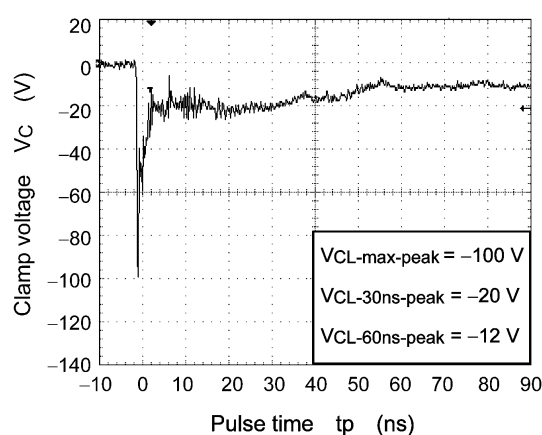
Fig. 10.2 -8 kV
