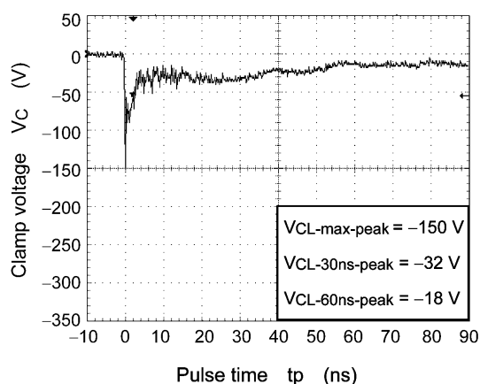
Fig. 10.4 -15 kV
