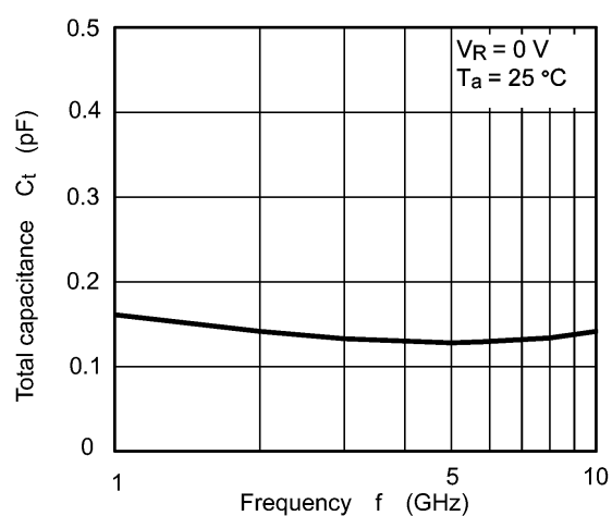
Fig. 7.4 C_t - f
