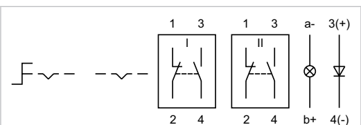
Wiring diagram 24
