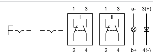
Wiring diagram 24
