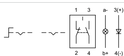
Wiring diagram 20
