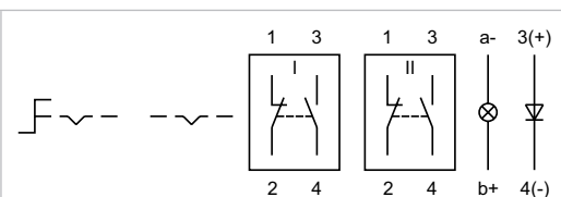
Wiring diagram 24
