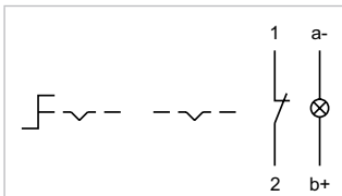
Wiring diagram 15
