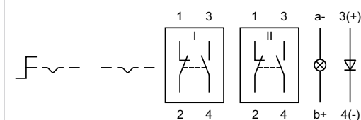
Wiring diagram 24
