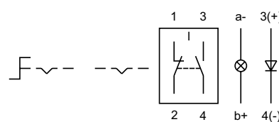
Wiring diagram 20
