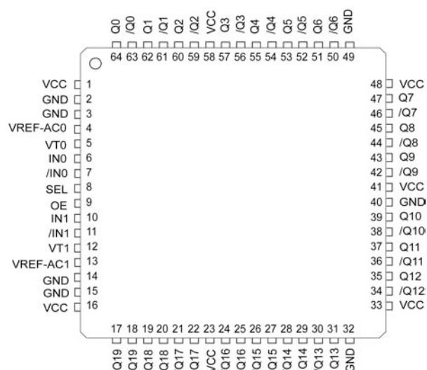
64-Pin EPAD-TQFP (H64-1)
