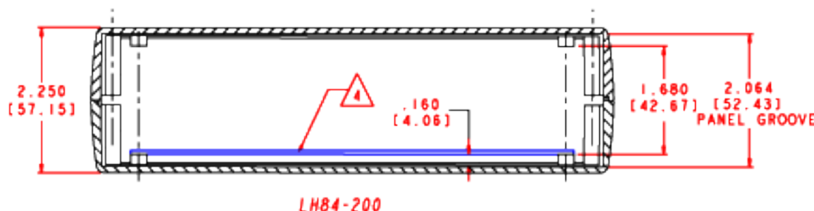
LH84-200 SECTION A-A
