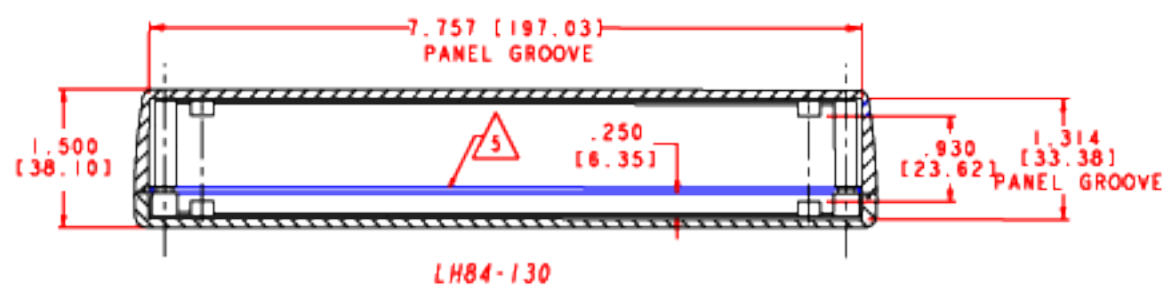
LH84-130 SECTION A-A
