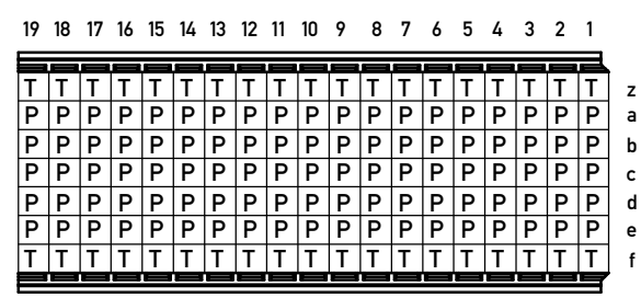
Bestückungsplan / contact layout
