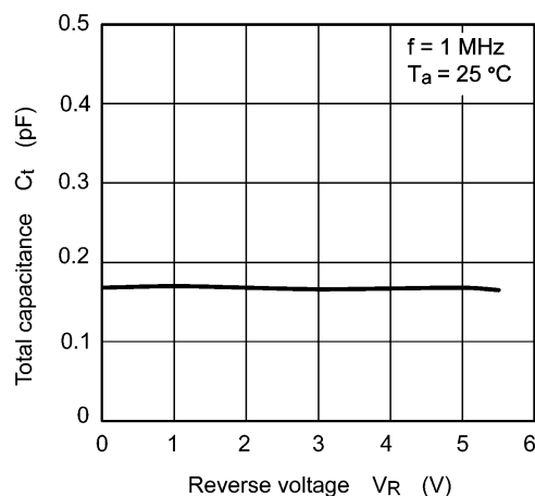
Fig. 9.3 C_t - V_R
