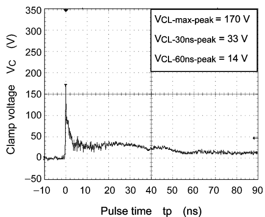
Fig. 6.1.3 +15 kV
