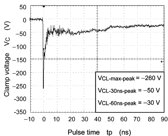
Fig. 6.1.4 -15 kV
