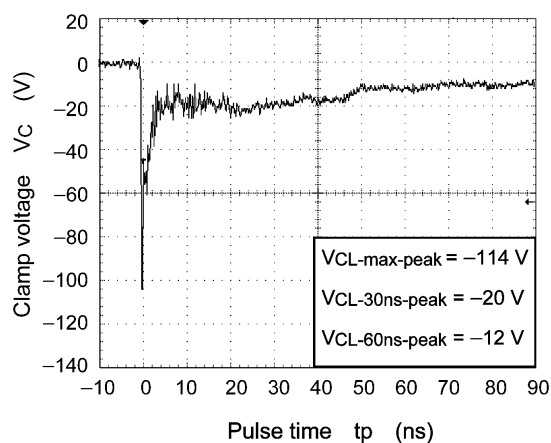
Fig. 6.1.2 -8 kV
