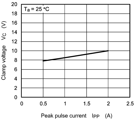
Fig. 6.3.1 V_C - I_{PP}
