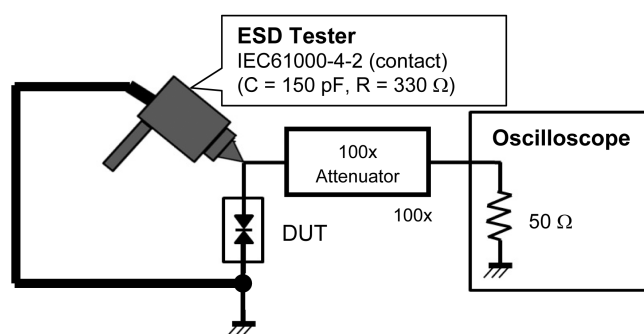
Fig. 6.1.5 IEC61000-4-2 (Contact)
