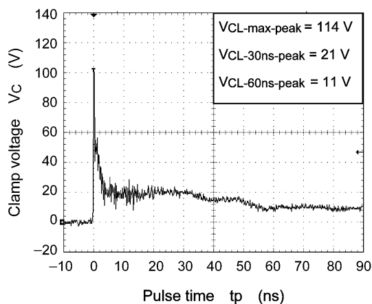
Fig. 6.1.1 +8 kV
