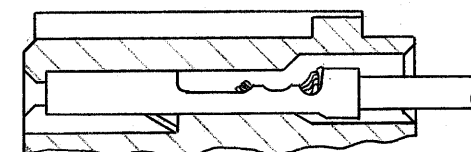
ファステニアストン接合状態 (FASTIN-FASTON MATING STATE)
