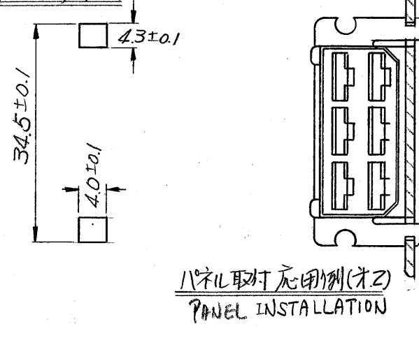
PANEL CUTTING DIMENSION パネル打抜寸法
