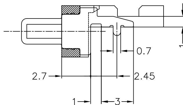
SECT."A"—"A" (SCALE:5-1)
