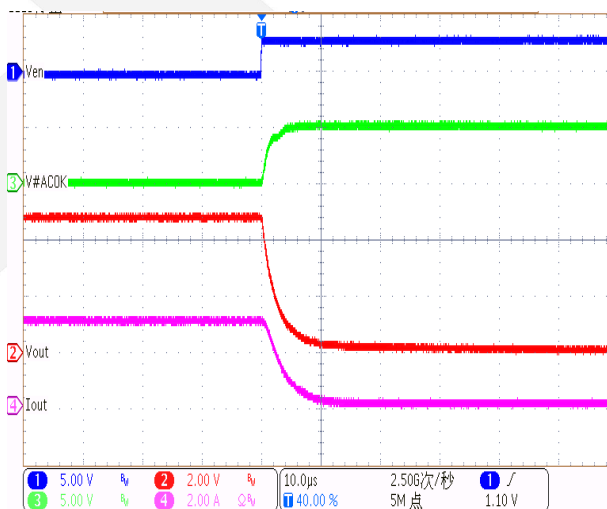
EN Power OFF ( V_{IN}=5V , R_{Load}=1.6ohm )
