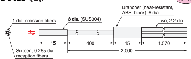
E32-D32L R25
