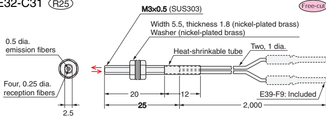
E32-C31 R25
