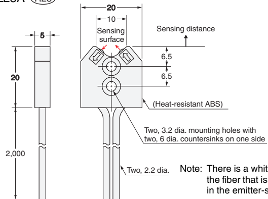
E32-L25A R25
