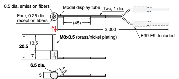
E32-C31N R
