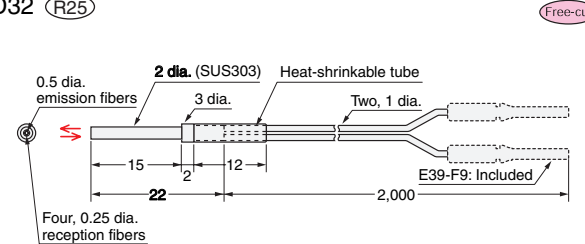
E32-D32 R25
