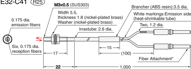
E32-C41 R25
