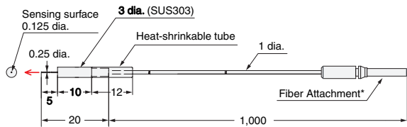
E32-T333-S5 R10
