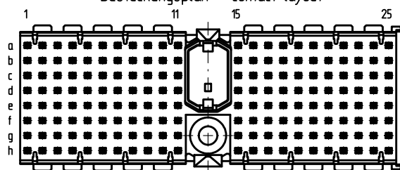
Bestückungsplan - contact layout
