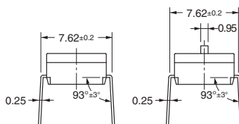
Flat Actuator
