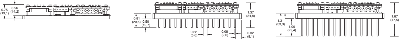
Coldplate
