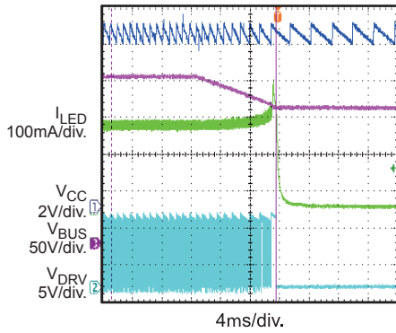
V_{BUS} Turn Off V_{IN} = 12.5V
