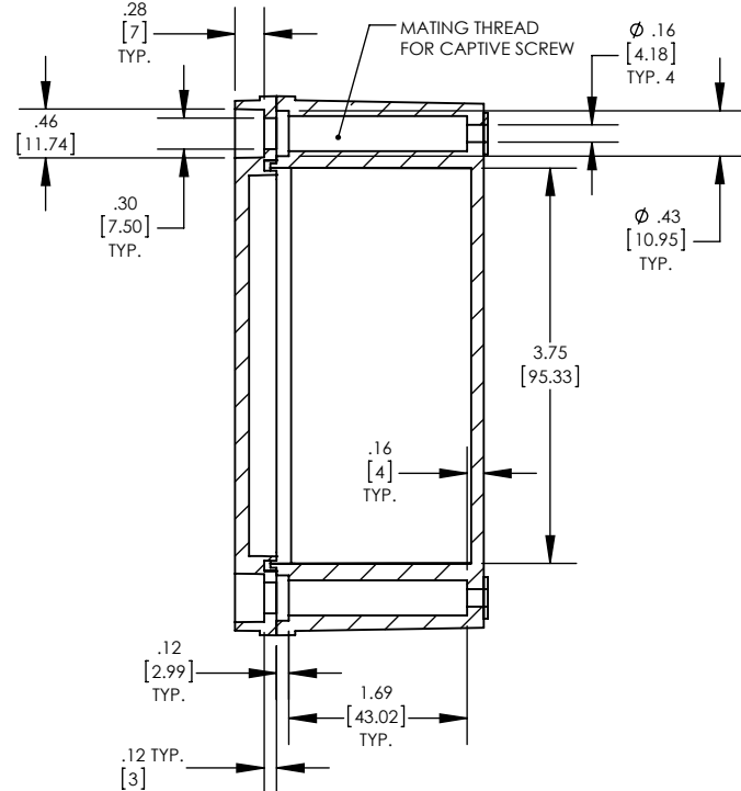
SECTION D-D
