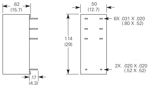
1 Pole 16A 2 Pole 8A 5mm
