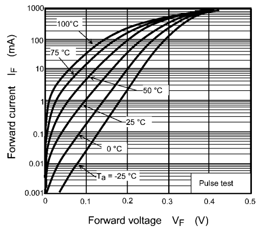
Fig. 9.1 I_F - V_F
