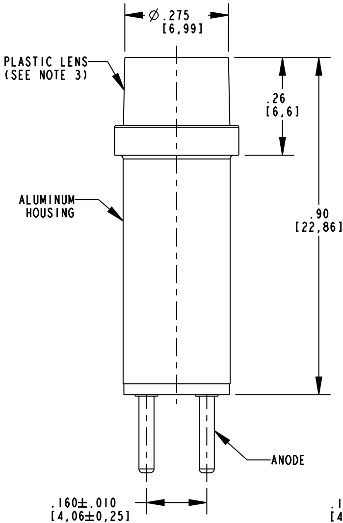
FIG. 1 (CYLINDRICAL LENS)
