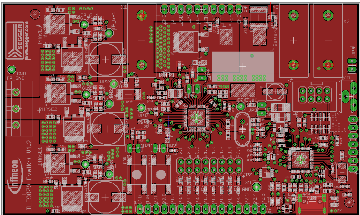
Top Layer
