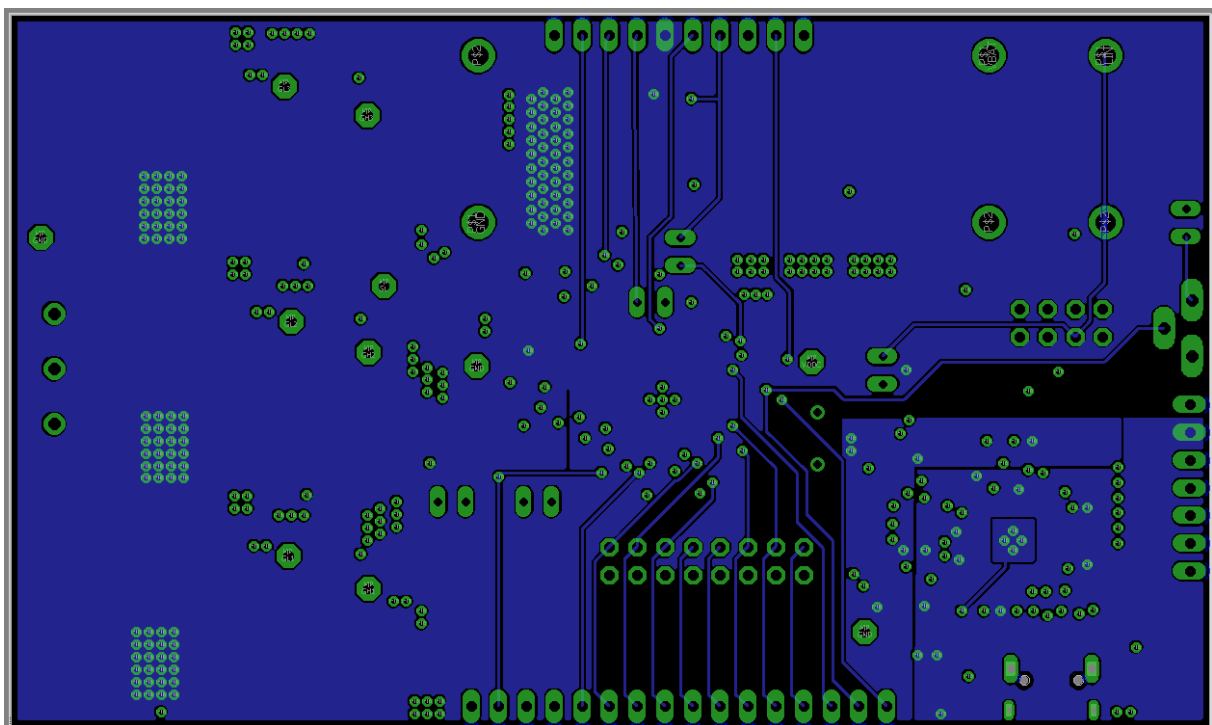
Bottom Layer
