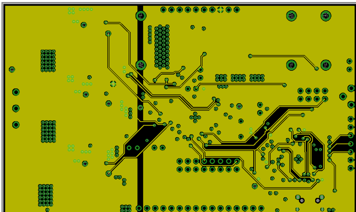
Layer 2
