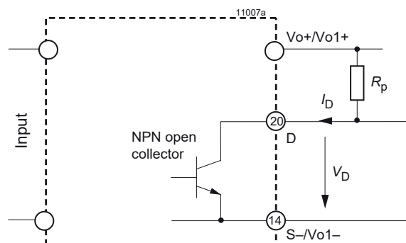
Fig. 36 Option D5 – DD: NPN output, V_D \leq 40 V , I_D \leq 2.5 \text{ mA}
