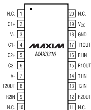
TSSOP
