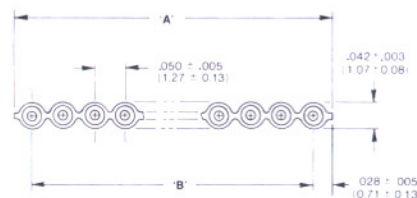
28 AWG SHOWN
