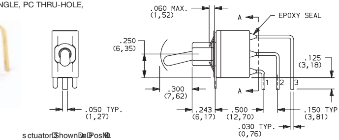
E101MD1AV2BE Vertical Actuation SPDT
