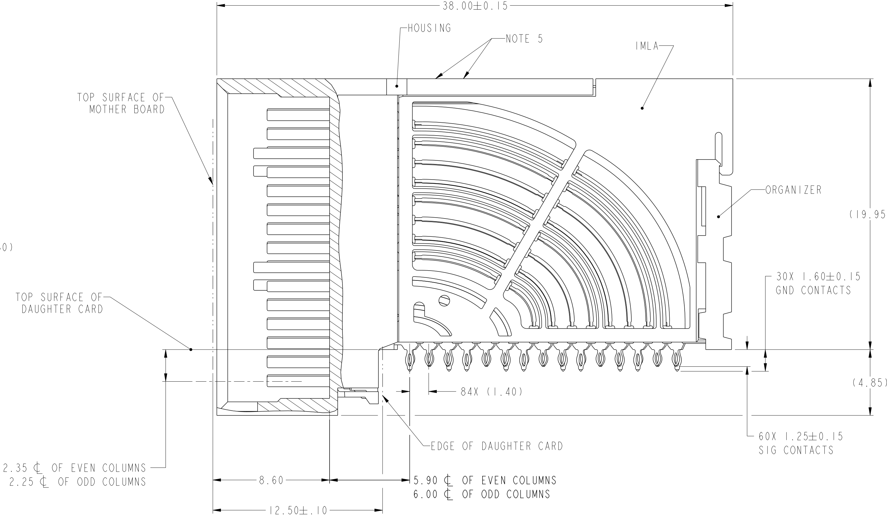
SECTION AA-AA
