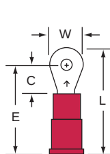
11-2S-P Stud Size Wire Range 2 22-18
